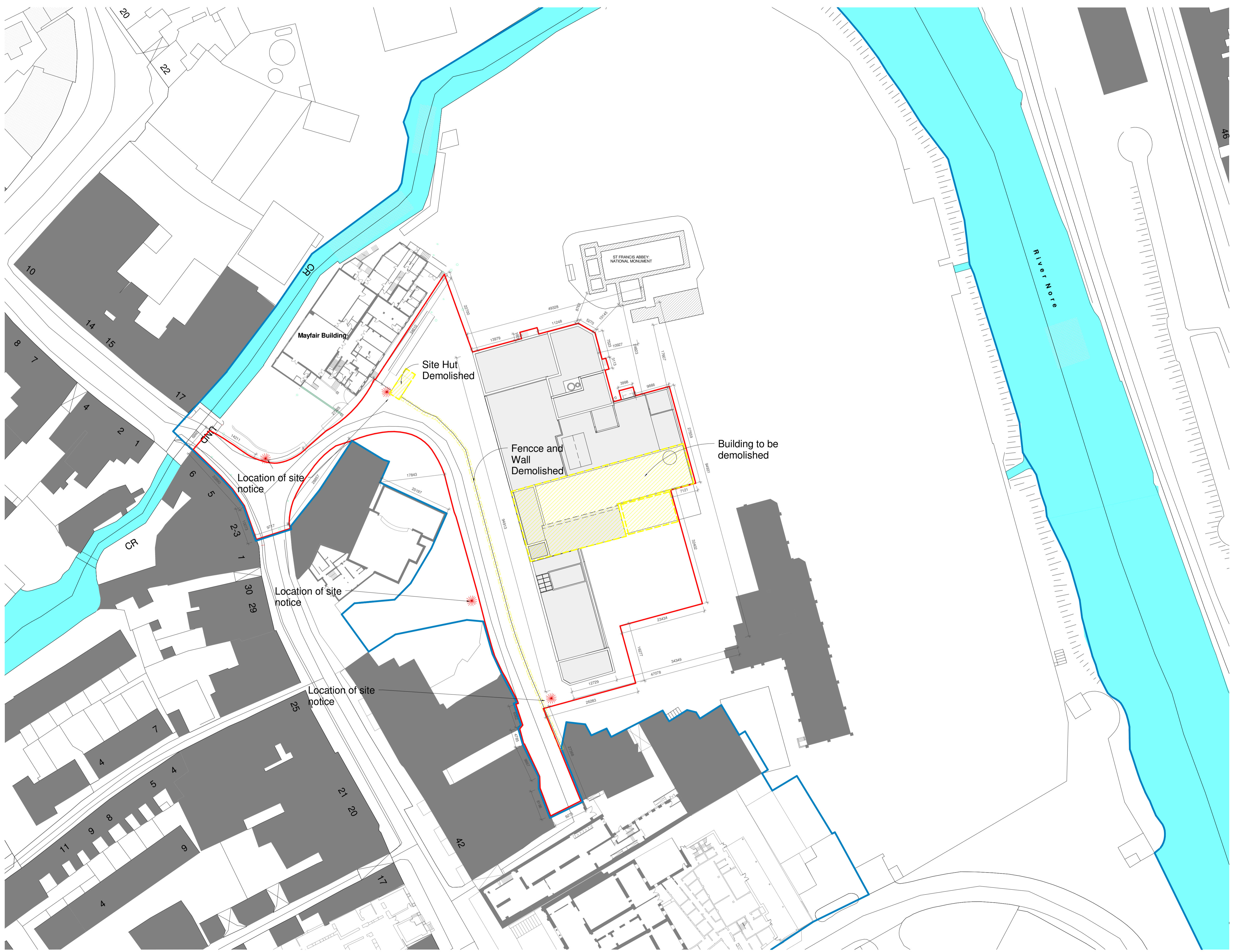
1 Site Plan Demolition 1 : 500
