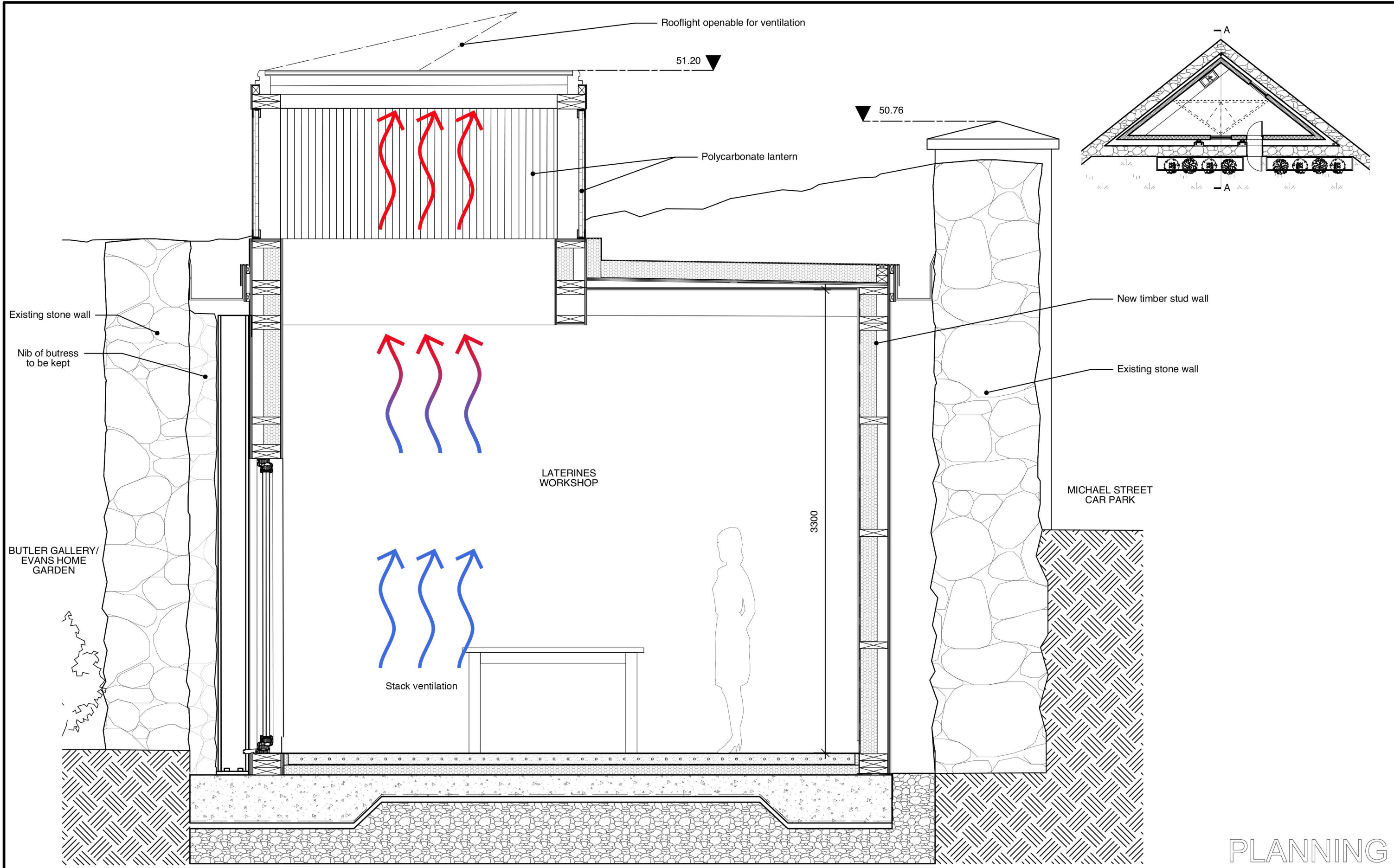
1 Section AA Scale: 1:25
