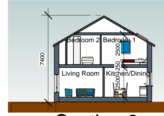
8 Section 2 1 : 200
