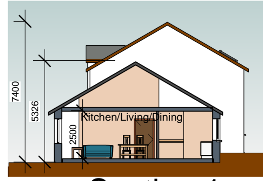
7 Section 1 1 : 200
