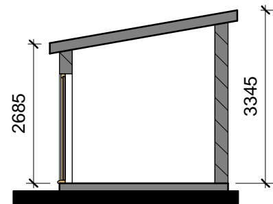
6 Section 1 : 100
